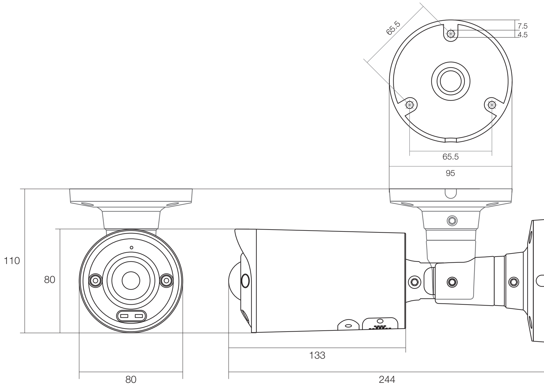
図名 4K 800万画素 PoE 対応 赤外線カメラ 図番 WTW-PRP240EA WIRELESS TSUKAMOTO CO., LTD
