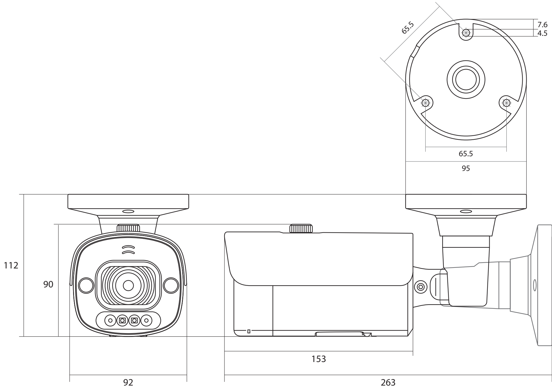
図名 4K 800万画素 PoE 対応 赤外線カメラ 図番 WTW-PRP26EA WIRELESS TSUKAMOTO CO., LTD
