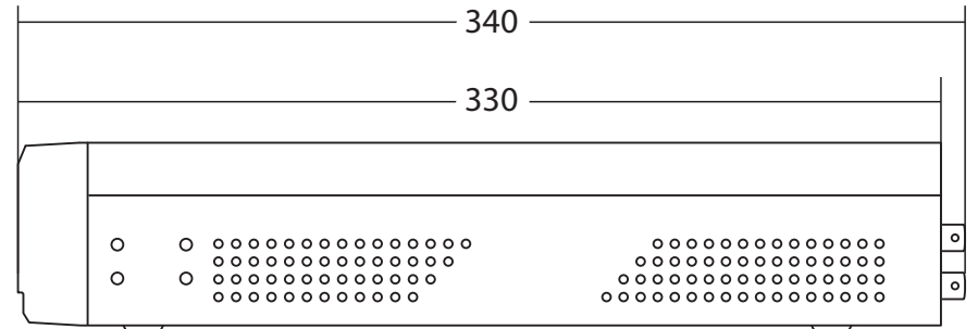
図名 500万画素 AHDシリーズ 32ch DVR 図番 WTW-DAP3332G
