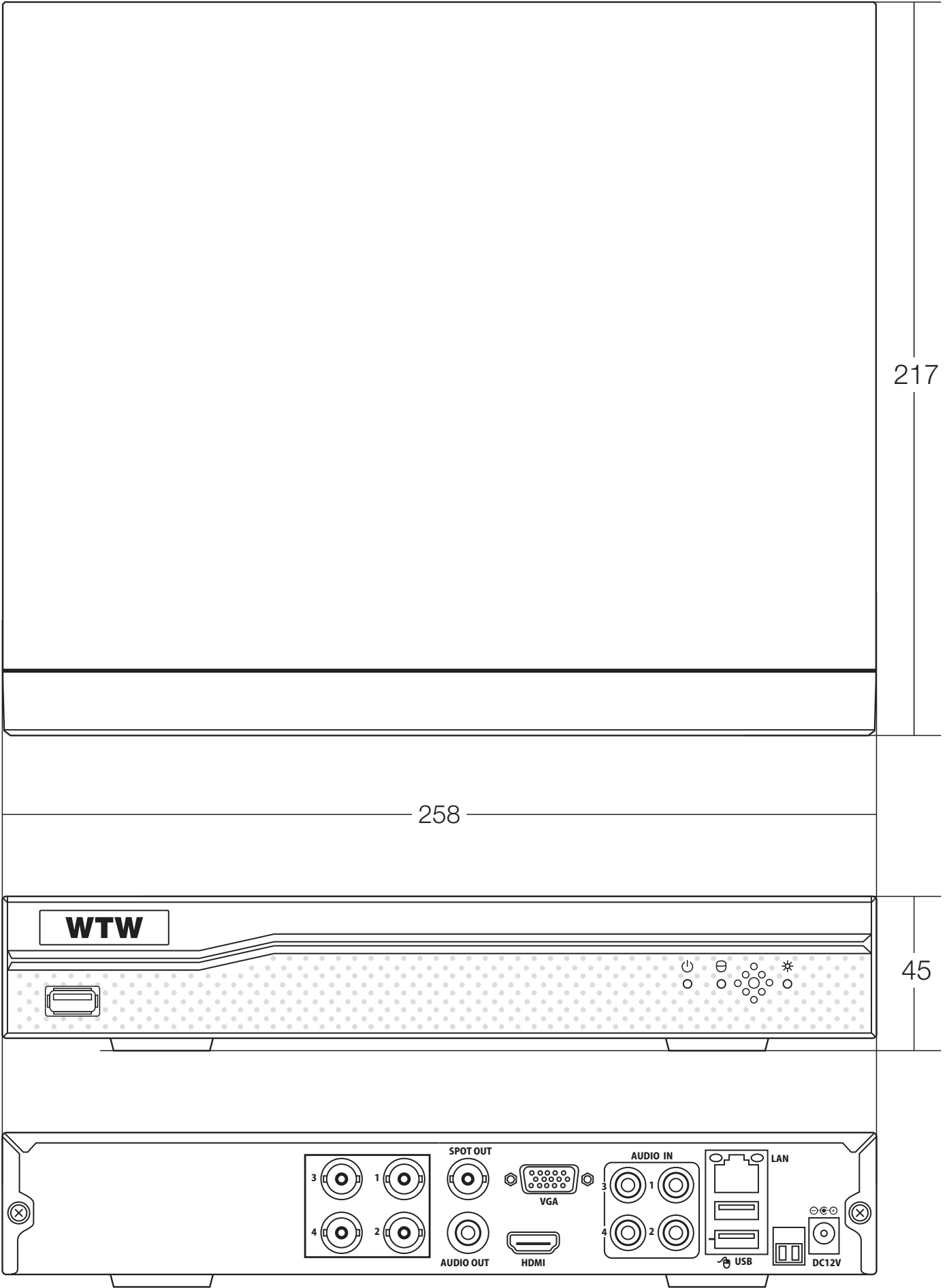
図名 4K 800万画素 AHDシリーズ 4ch DVR 図番 WTW-DA8004E WIRELESS TSUKAMOTO CO., LTD
