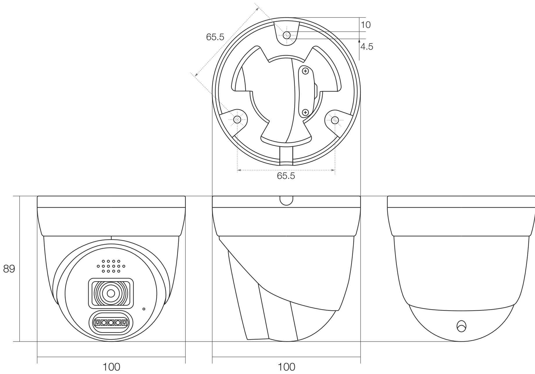
図名 PoE対応ドーム型カメラ 図番 WTW-PDRP50HA WIRELESS TSUKAMOTO CO., LTD
