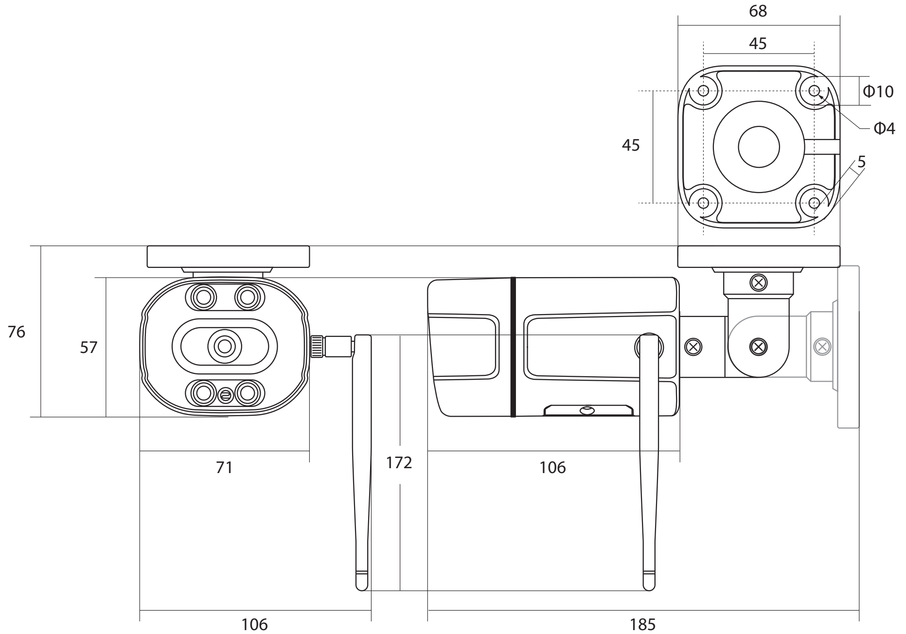
図名 300万画素 WiFi カメラ 図番 WTW-EGR2319SPBX WIRELESS TSUKAMOTO CO., LTD
