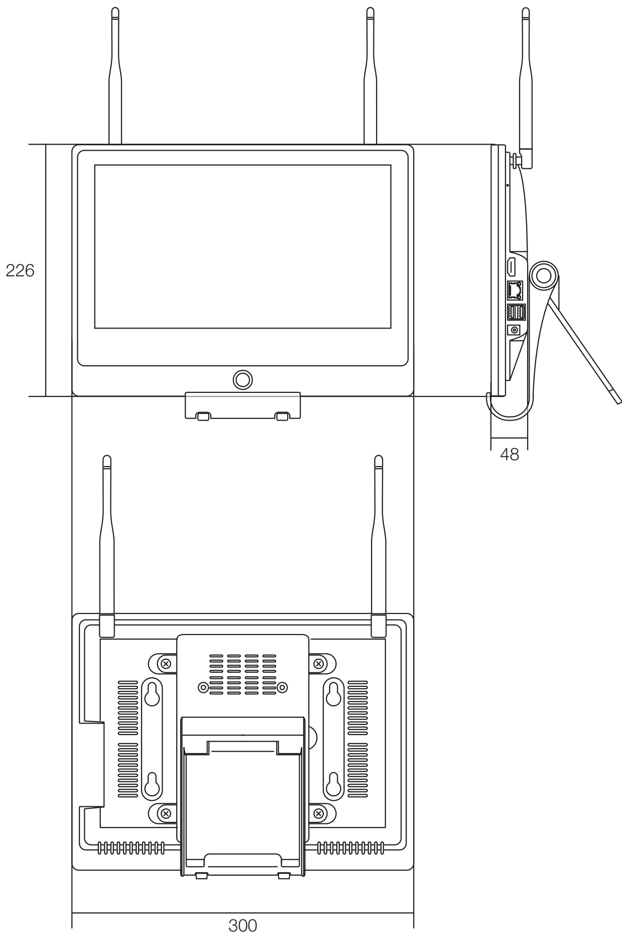
図名 IPカメラシリーズ用 10CHデジタルレコーダー 図番 WTW-EG2610WHA WIRELESS TSUKAMOTO CO., LTD
