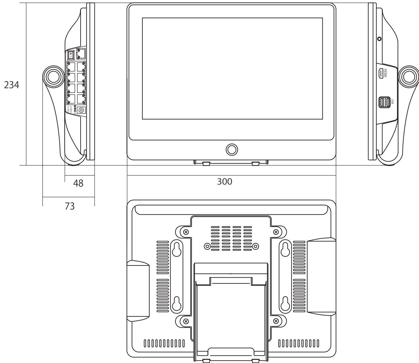
図名 XPoE 8ch対応 12インチモニター内蔵 (NVR) 図番 WTW-ENV279GPL
